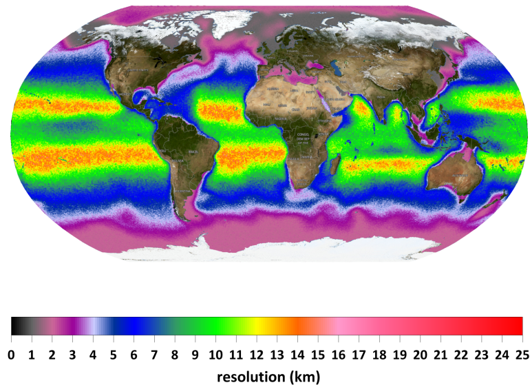
Fig.1 FESOM2-ER resolution
